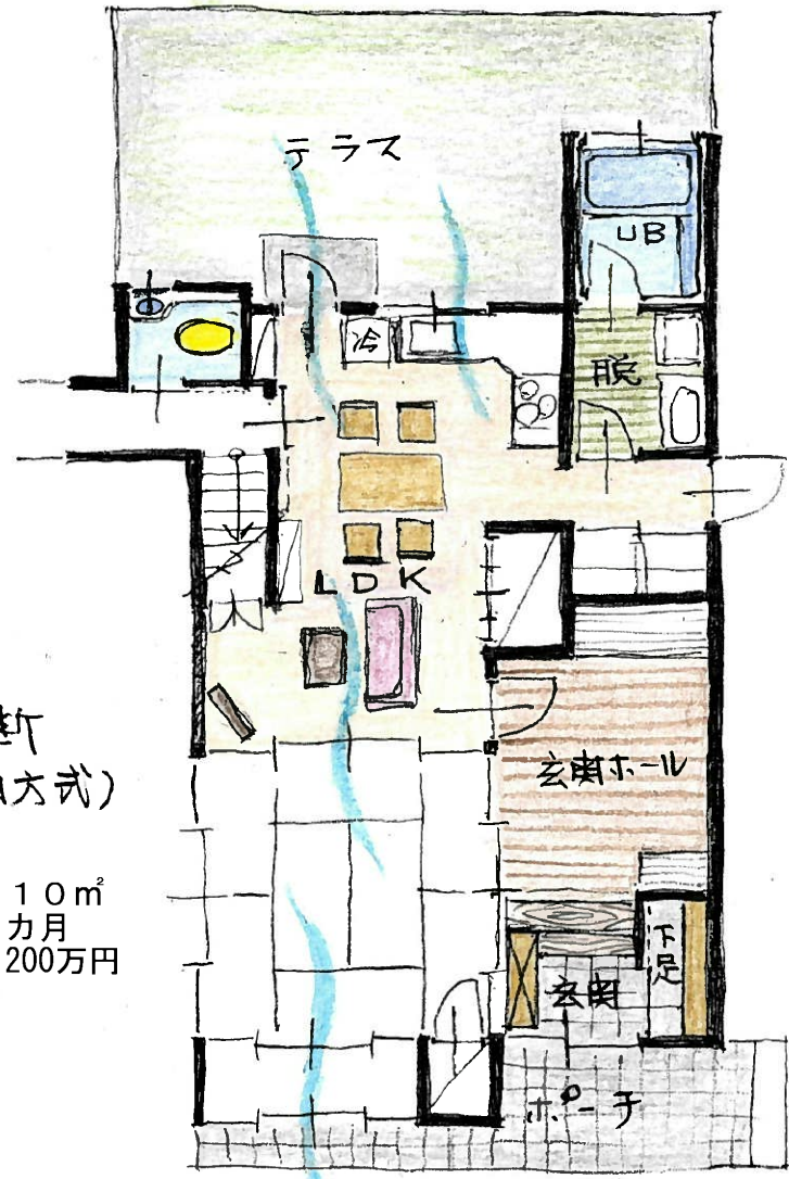
(改修後平面図)
